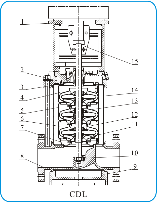
截面图 CDL,CDLF32,42,65,85
