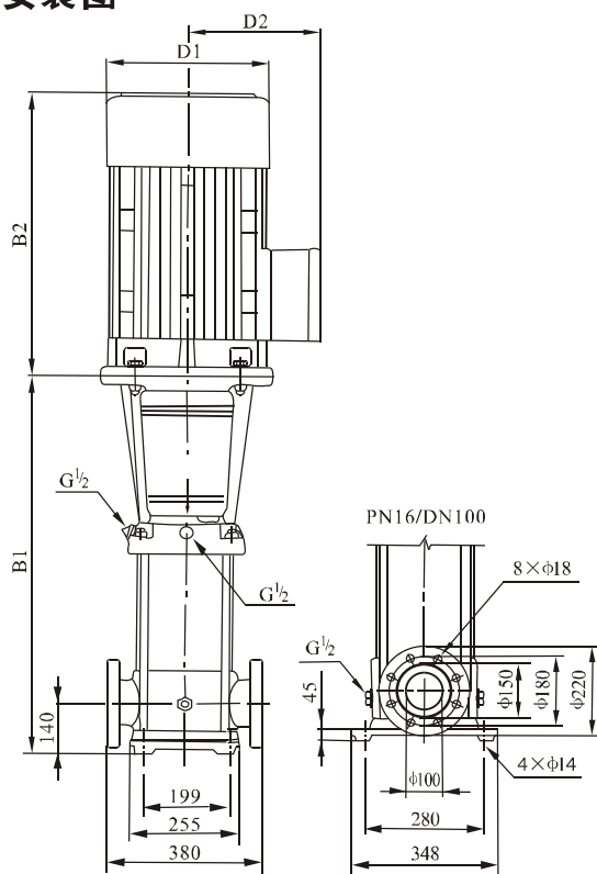
安装图
